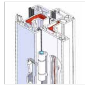
FERRAGE TRIPLE BROCHE
