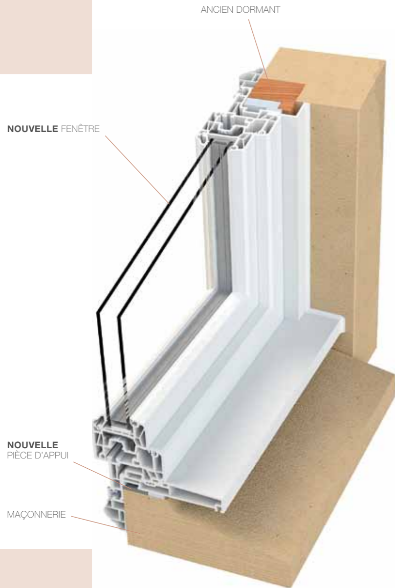
POSE EN RÉNOVATION AVEC DÉPOSE DE L'APPUI
